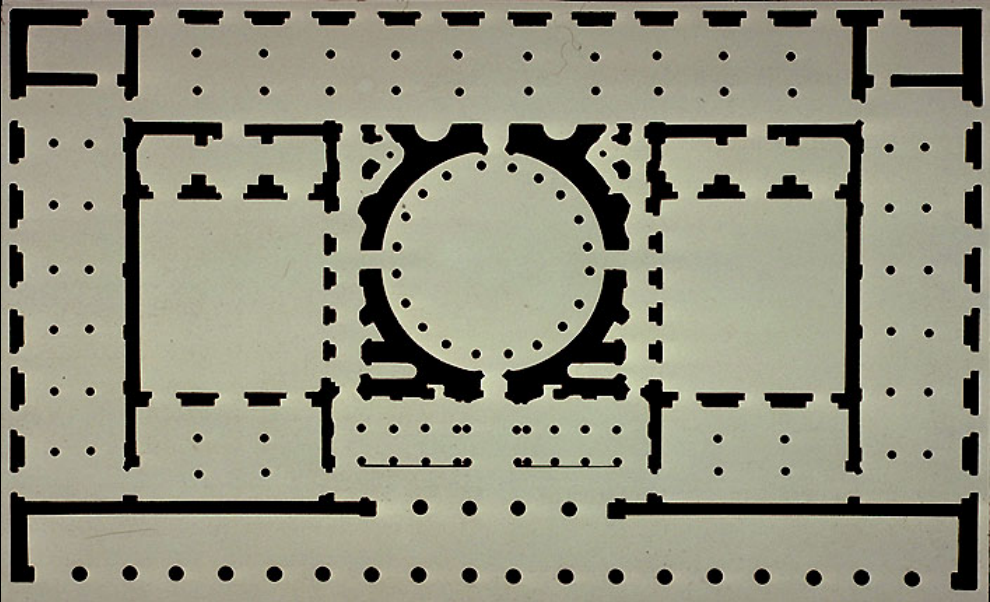
Schinkel, Altes Museum, do Sammlung Architektonischer Entwürfe , Prancha 38, det. Primeiro piso
