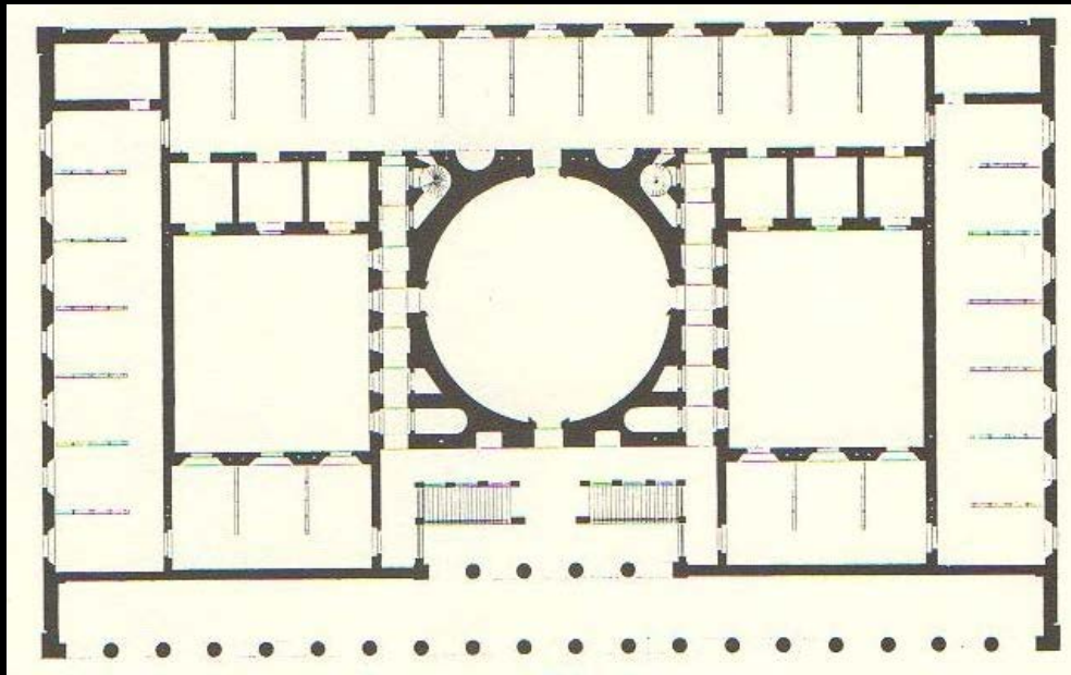
Schinkel, Altes Museum, do Sammlung Architektonischer Entwürfe , Prancha 38, det. segundo piso
